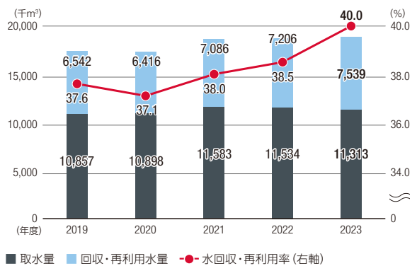
生産拠点の取水量、回収・再利用水量、水回収・再利用率
